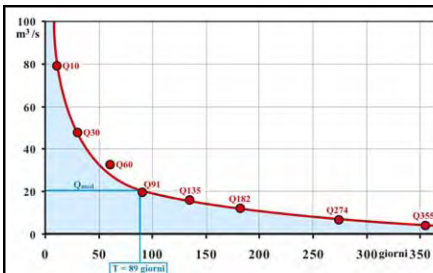
Fig. 4 - Curva di durata delle portate dello Stura di Lanzo a Lanzo. ( S = 582 \text{ km}^2 ). Periodo di osservazione 1930÷1943 e 1946÷1981 (50 anni). Portata media annua ( Q_{med} = 20,2 \text{ m}^3/\text{s} ) (portate pari o superiori sono disponibili in alveo per un tempo T = 89 giorni , 24 % dell'anno) per un volume complessivo medio annuo V_{med} = 6,37 \cdot 10^8 \text{ m}^3/\text{anno} ). Da: PE-ROSINO, 2005.
